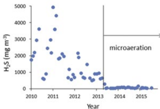
Rysunek: Stężenie H 2 S w gazie osadowym oczyszczalni ścieków przed i po wdrożeniu Mikroaeracji przy użyciu powietrza.
